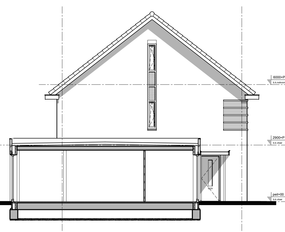
doorsnede / zijgevel type B-basis
